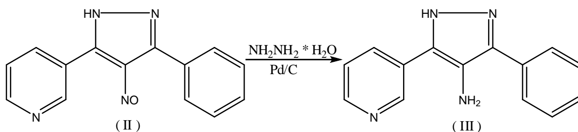
Рис.2. Синтез 3(5)-фенил-4-амино-5(3)-пиридин-3-ил-1H-пиразола
