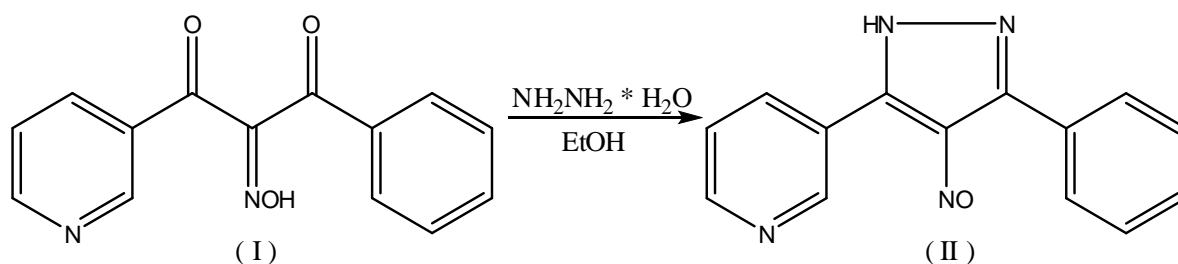
Рис.1. Синтез 3(5)-фенил-4-нитрозо-5(3)-пиридин-3-ил-1H-пиразола
